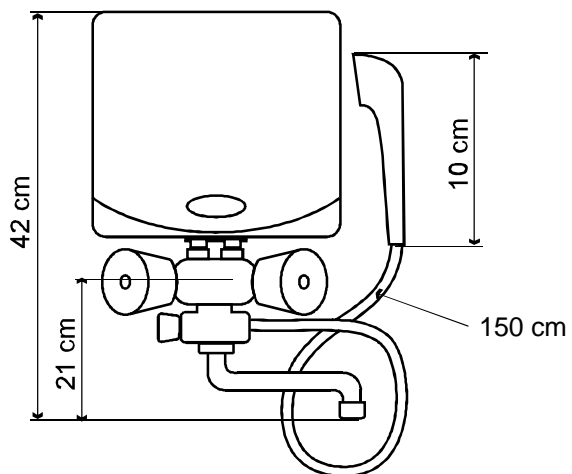
model kombinovaný
